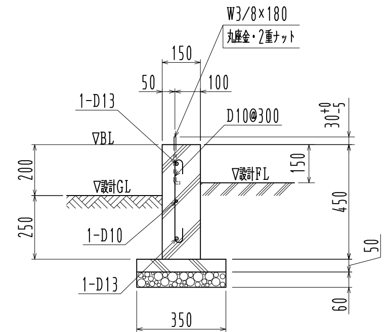
FG 1断面図 1/15
