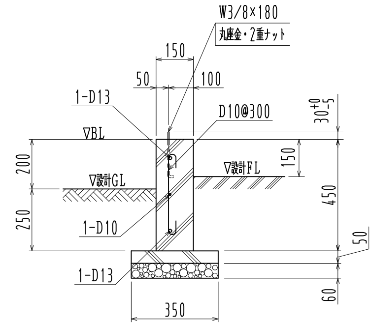
FG 1断面図 1/15
